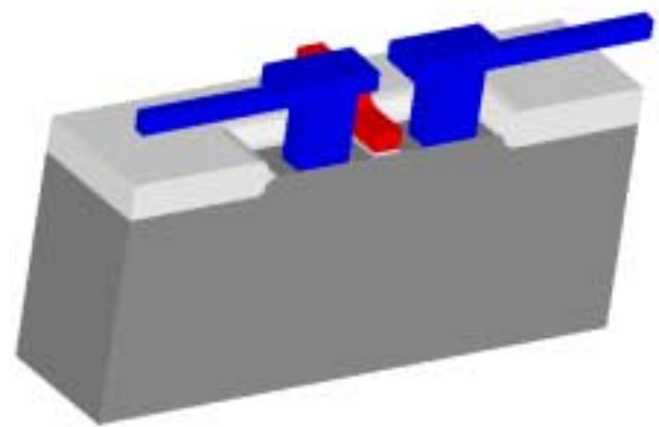
Silicon MOSFET
